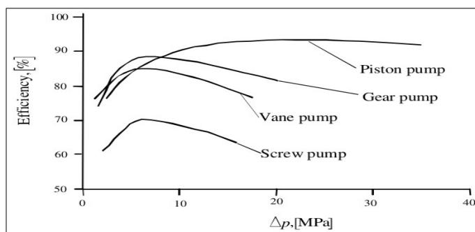
Gráfico 1 - Desempenho de diferentes tipos de bombas hidráulicas Fonte: Minav et al (2007)
