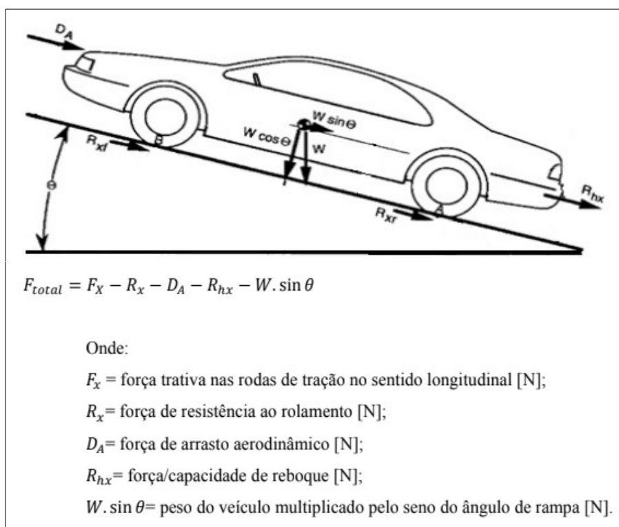
Figura 1 - Forças atuantes no movimento veicular (GILLESPIE, 1992)
